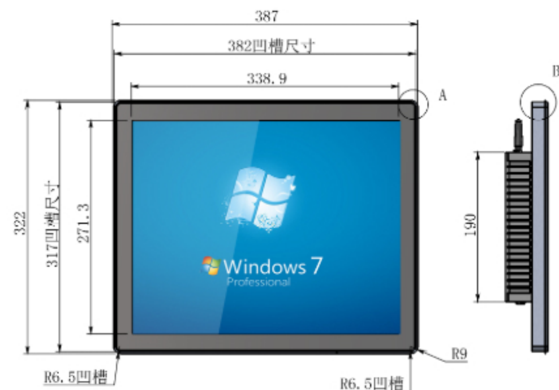
面框边角尺寸图 面框深度尺寸图
