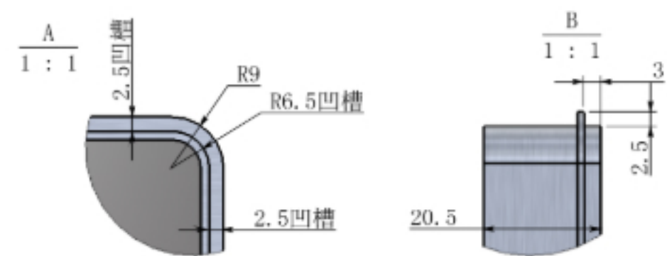
面框边角尺寸图 面框深度尺寸图
