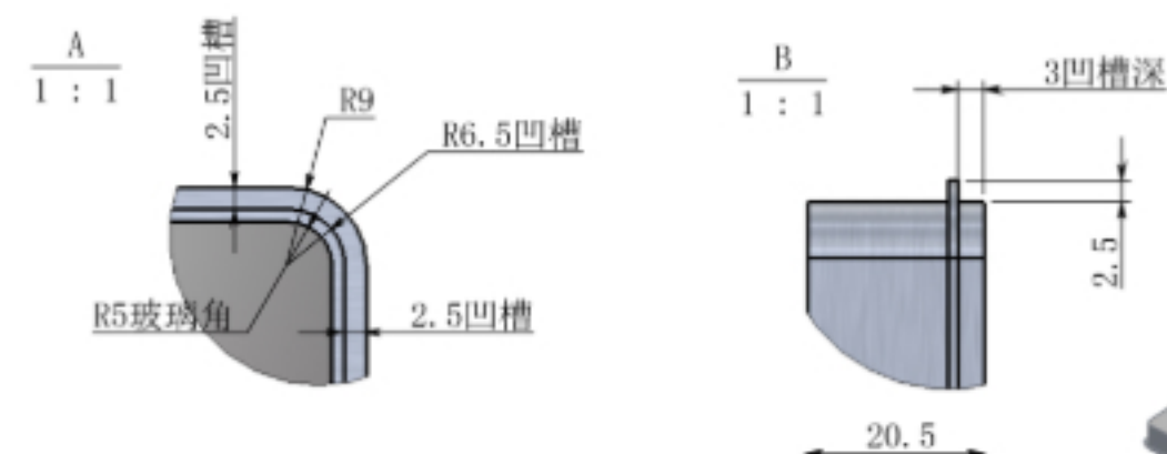
面框边角尺寸图 面框深度尺寸图
