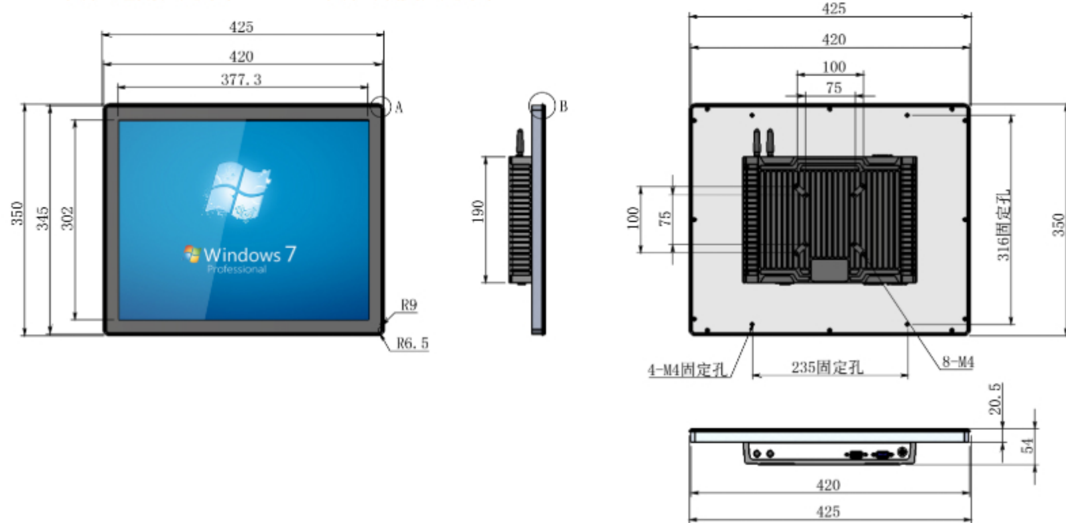
面框边角尺寸图
