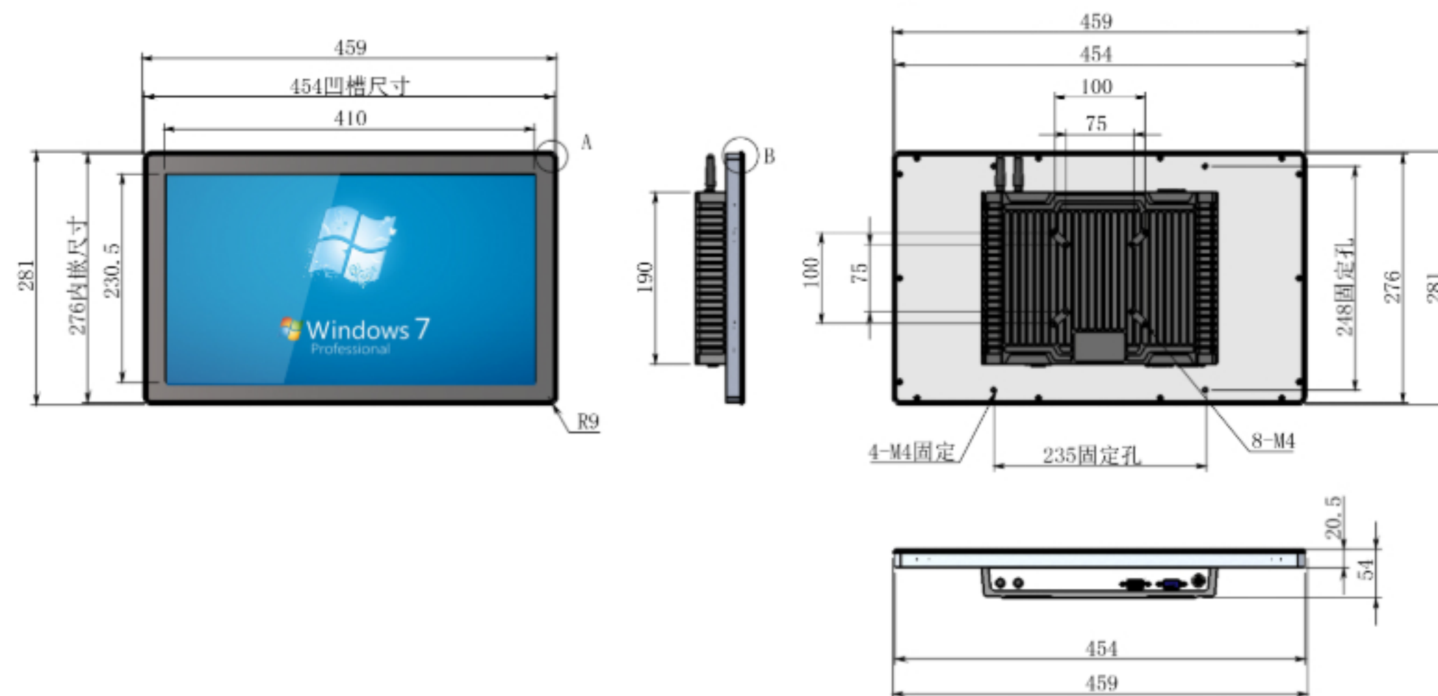
面框边角尺寸图 面框深度尺寸图
